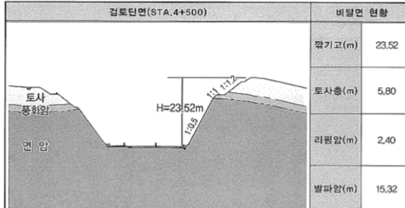
마. 깎기8구간
